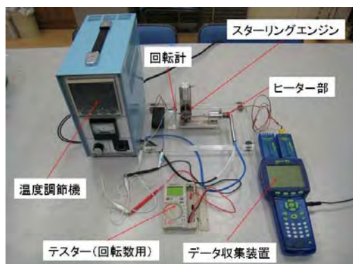
図1. 装置外観
