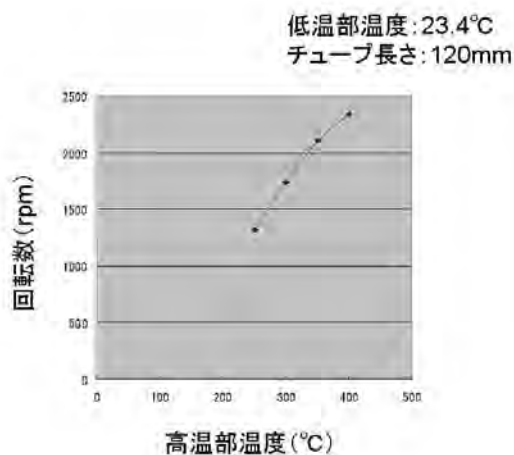
図6. 高温部温度－エンジン回転数
