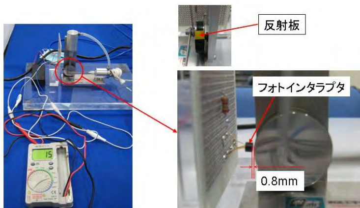
図 3. 回転計部分
