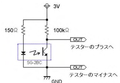
図 4. 回路図
